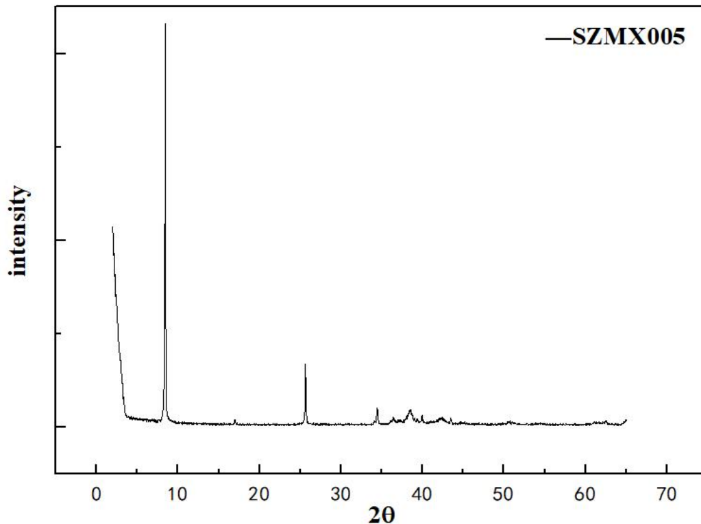
图 3 碳化钼 Mo 2 C (MXene) 多层纳米片的 XRD 图 Fig.3 XRD pattern of Mo 2 C (MXene) multilayer nanoflake
